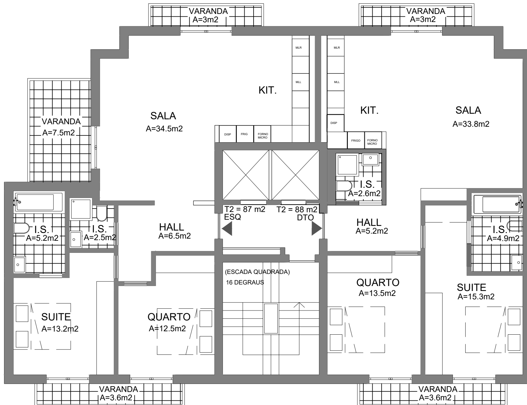
PLANTA DO PISO TIPO (1 a 11)
